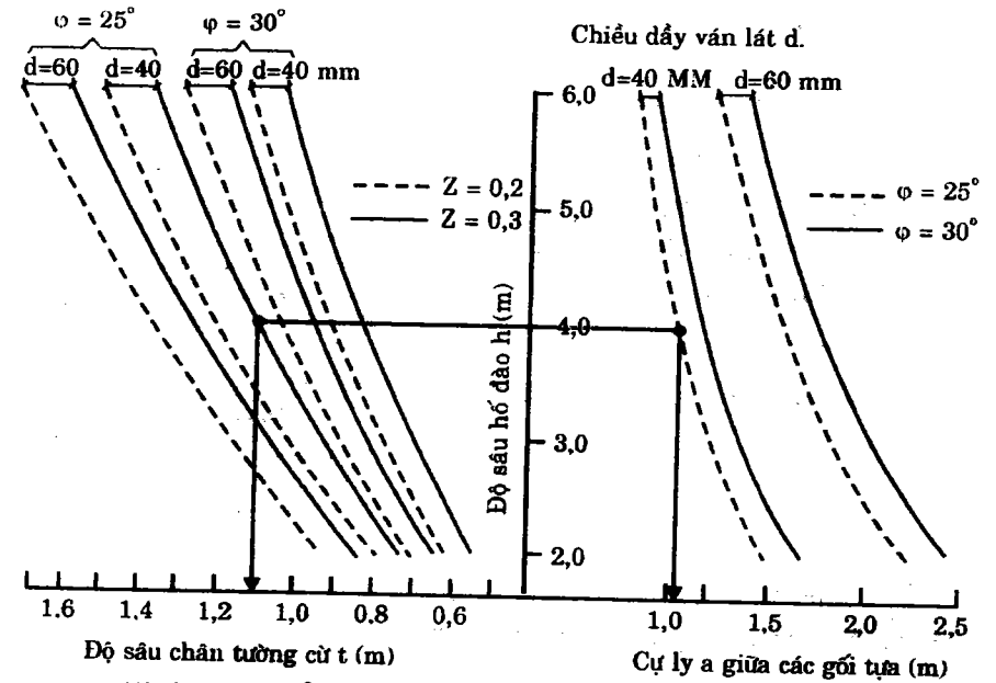
Hình 1-14. Biểu đồ để xác định các thông số của tường cừ có một gối tựa A.
