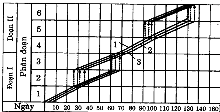
Hình 3-15 - Tiến độ dây chuyền lắp ghép kết cấu công trình. 1 - lắp kết cấu bê tông và kết cấu thép; 2 - hàn mối nối; 3 - gắn vữa mối nối và mạch lắp ghép.
