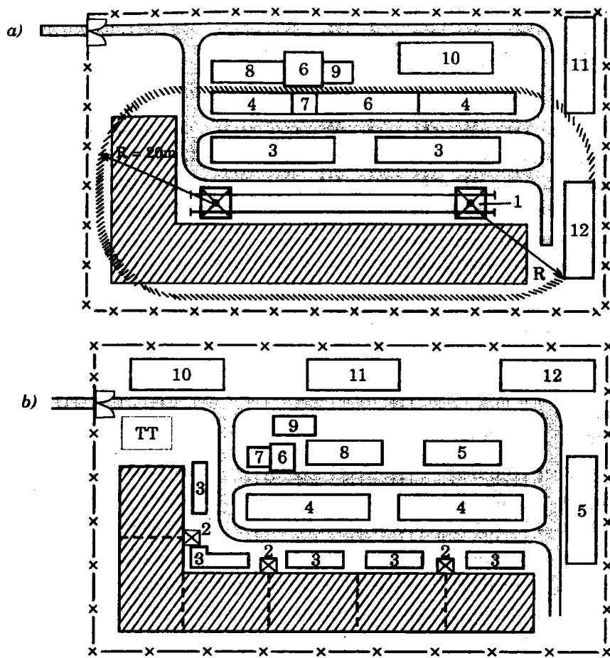
Hình 5-3: Tổng bình đồ thi công một ngôi nhà ở nhiều tầng bằng gạch a) Trường hợp sử dụng cần trục tháp b) Trường hợp sử dụng các máy thăng tải cố định
