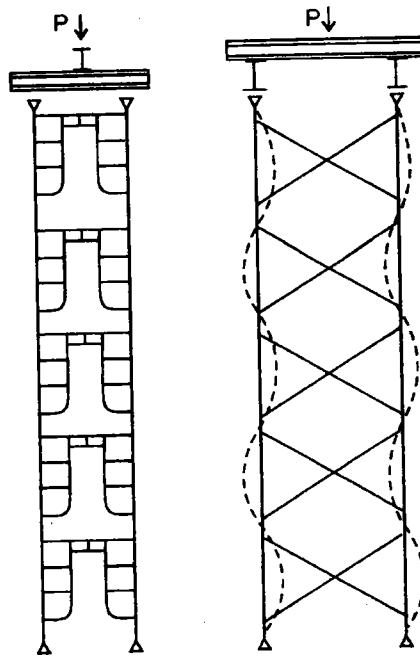
TẢI TRỌNG CHO PHÉP CỦA KHUNG KHÔNG GIAN P = 200\text{kN}
