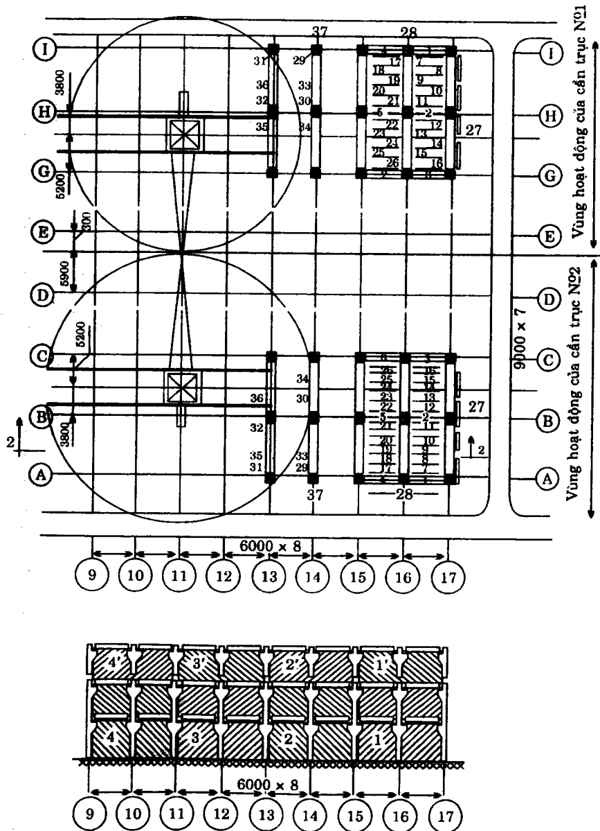
Hình 3-14 - Trình tự lắp ghép kết cấu trong phân đoạn 2 và 3.
