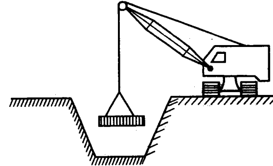
Hình 1-7: Gia cố nền bằng đầm chày.
