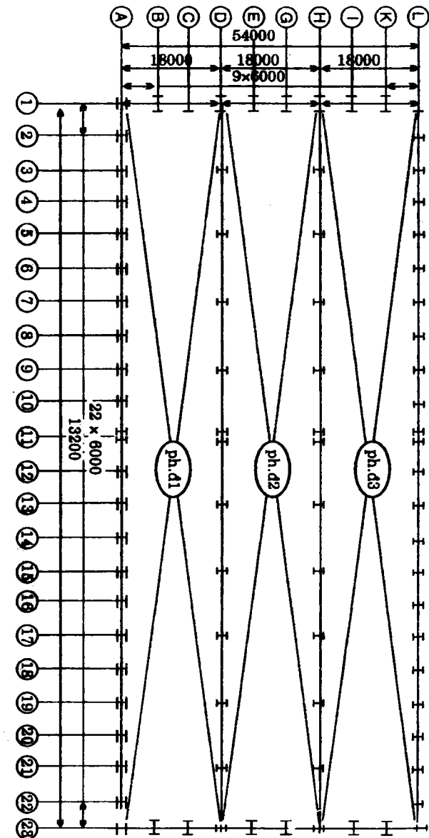
Hình 3-9 - Phân chia nhà xưởng thành những phân đoạn lắp ghép.
