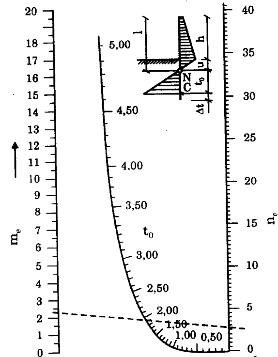
Hình 1-16. Biểu đồ để xác định độ ngập t_0 trong đất nền của tường cừ
