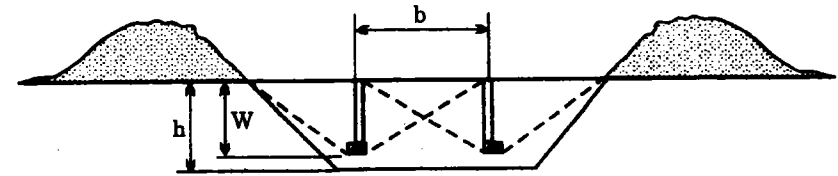
Hình 1-11: Nổ mìn để đào hồ nước
