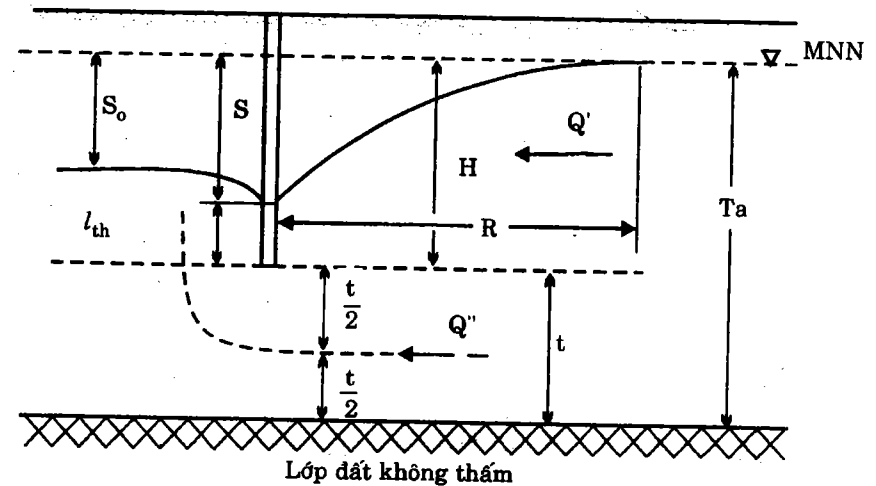
Hình 1-9: Sơ đồ tính lượng nước ngầm thấm vào giếng lọc.
