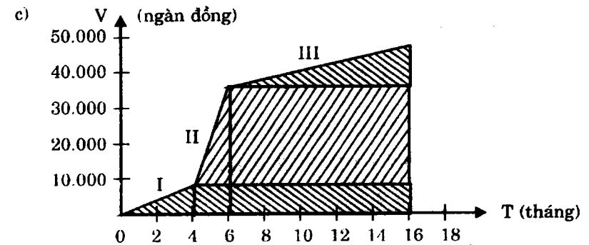
Hình 4-3: Các sơ đồ phân phối vốn đầu tư a) Phương án lắp ghép 1; b) Phương án lắp ghép 2 và 3; c) Phương án lắp ghép 4;
