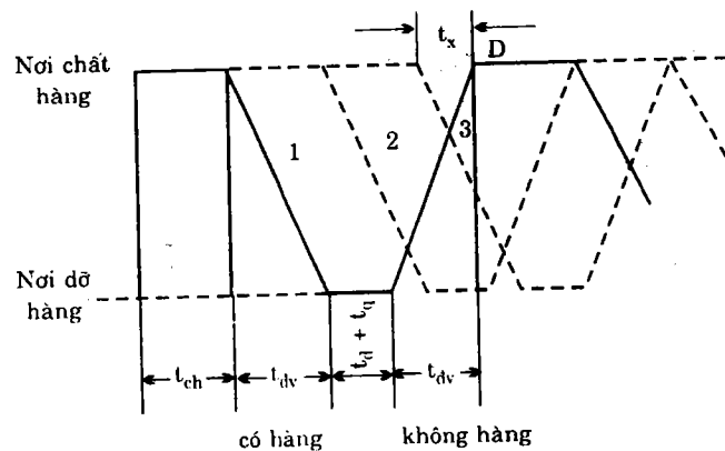
Hình 1-5: Đồ thị vận động của các xe tải. 1. xe thứ nhất; 2. xe thứ hai; 3. xe thứ ba.
