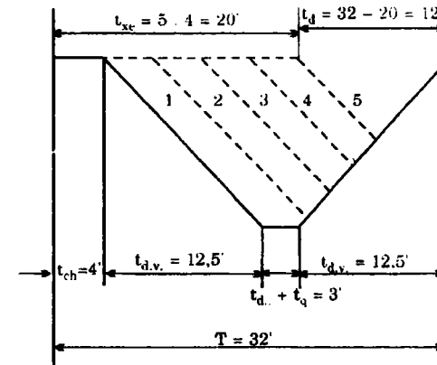
Hình 1-6: Đồ thị vận động của các xe ô tô tải.
