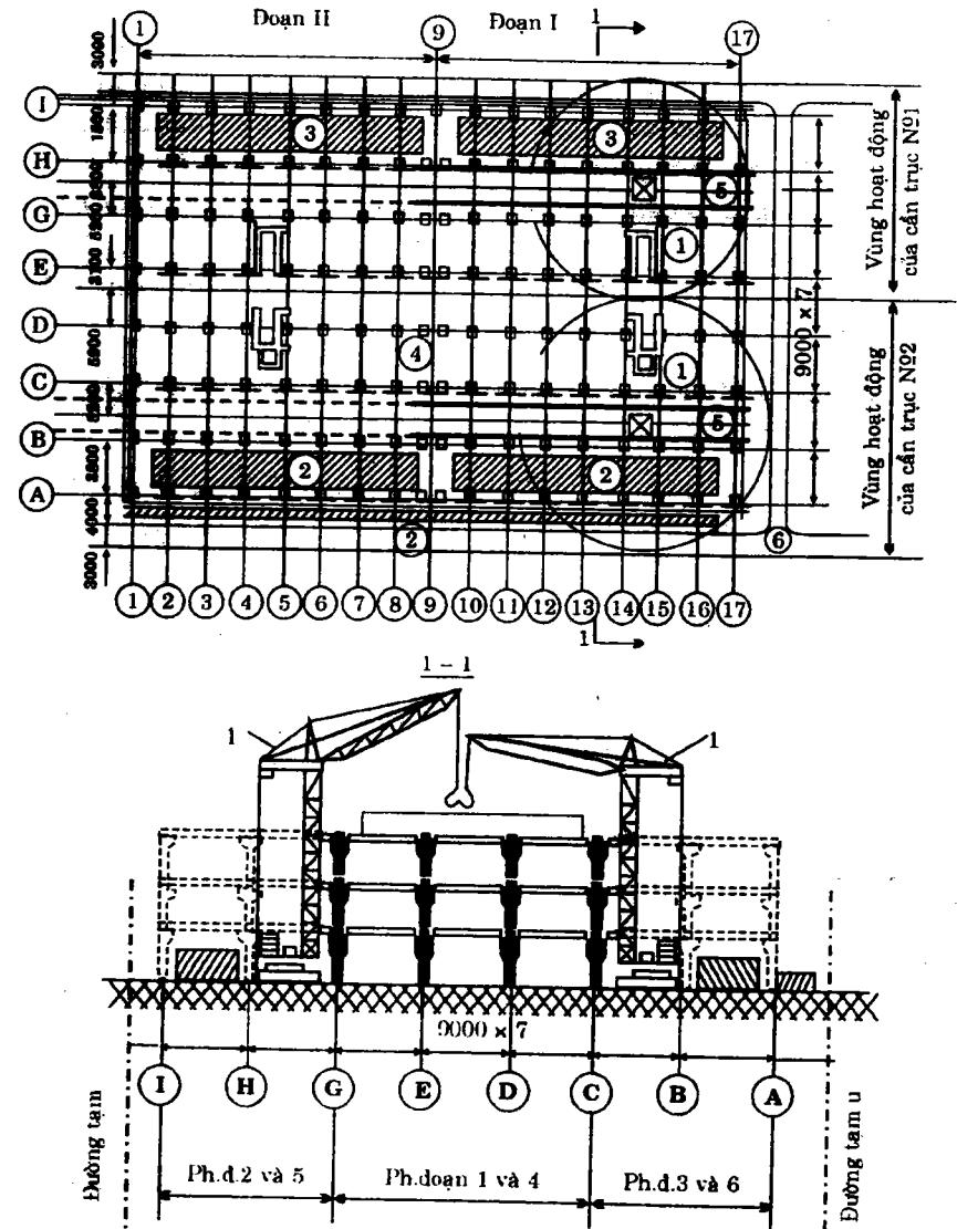
Hình 3-12 - Sơ đồ bố trí các cần trục lắp ghép. 1 - cần trục tháp; 2 và 3 - bãi chứa cấu kiện nằm trong tầm với của cần trục; 4 - Mặt bằng lắp ghép nhà máy; 5 - Đường cần trục tháp; 6 - Đường sá tiếp vận cấu kiện.
